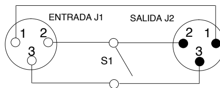
DIAGRAMA DE ALAMBADO PARA INTERRUPTOR FIGURA 6
