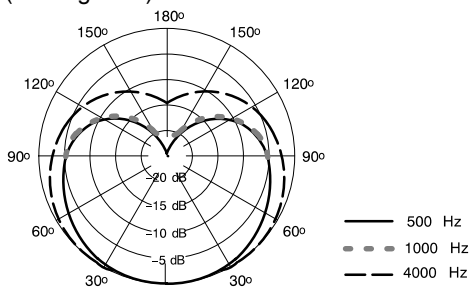
COURBE DE DIRECTIVITÉ TYPIQUE FIGURE 3
