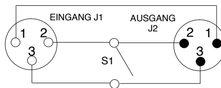
SCHALTPLAN FÜR EIN/AUS-SCHALTER ABBILDUNG 6
