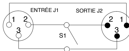
SCHÉMA DE CÂBLAGE DE L'INTERRUPTEUR MARCHE-ARRÊT FIGURE 6
