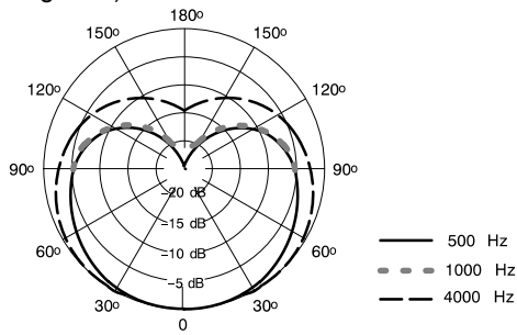
PATRÓN POLAR TÍPICO FIGURA 3
