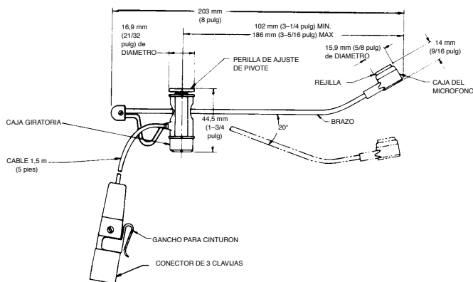
DIMENSIONES DEL SM10A Y CINTA PARA CABEZA FIGURA 5
