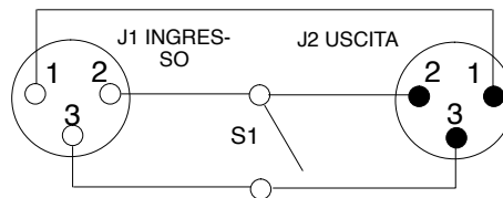
SCHEMA CIRCUITALE DELL'INTERRUPTORE DI ALIMENTAZIONE FIGURA 6
