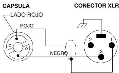
DIAGRAMA DE ALAMBRADO DEL SM10A FIGURA 4
