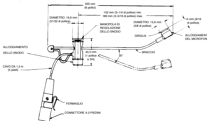
DIMENSIONI DEL GRUPPO SM10A-SUPPORTO FIGURA 5
