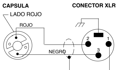
DIAGRAMA DE ALAMBADO DEL SM10A FIGURA 4
