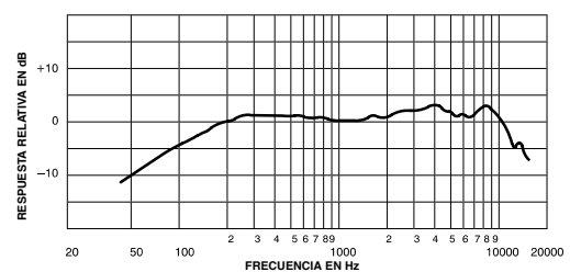
RESPUESTA DE FRECUENCIA TÍPICA FIGURA 2
