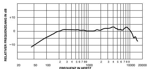
TYPISCHER FREQUENZGANG
