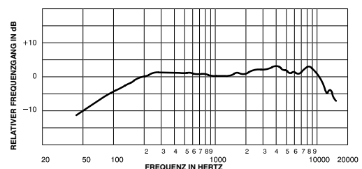
TYPISCHER FREQUENZGANG
