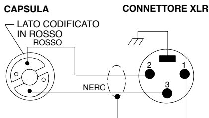
SCHEMA CIRCUITALE DEL MODELLO SM10A FIGURA 4
