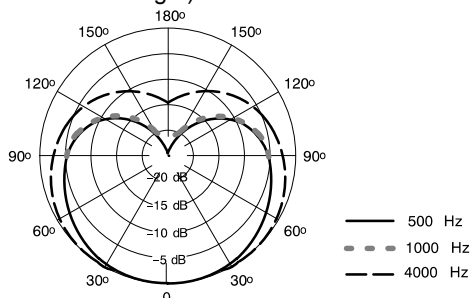
TYPISCHE RICHTCHARAKTERISTIK ABBILDUNG 3
