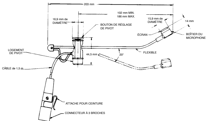
DIMENSIONS DE L'ENSEMBLE SM10A ET SERRE-TÊTE FIGURE 5
